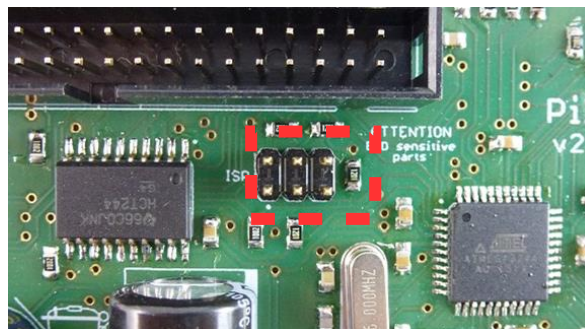
Abbildung 48: Steckverbinder - In-System-Programming (ISP)
