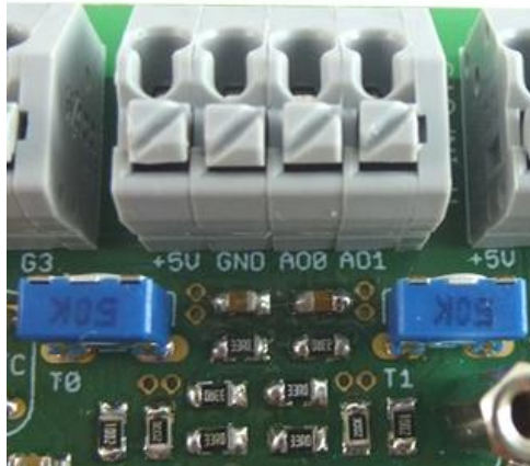
Abbildung 68: Anschlussleiste - analoge Ausgänge
