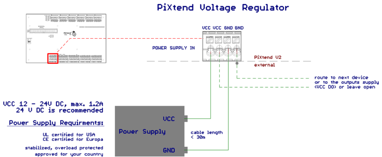
Abbildung 40: Prinzip-Schaltbild: Anschluss der Hauptversorgung
