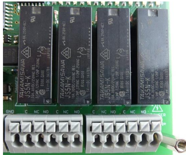
Abbildung 57: Anschlussleisten - Relais
