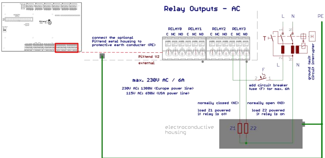
Abbildung 59: Prinzip-Schaltbild: Anschluss der Relais (Wechselspannung)
