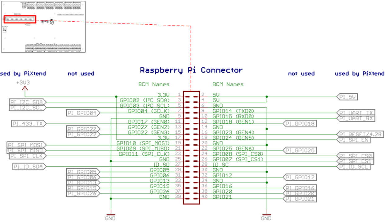
Abbildung 42: Prinzip-Schaltbild: Verbindung zwischen Raspberry Pi und PiXtend V2 -S-
