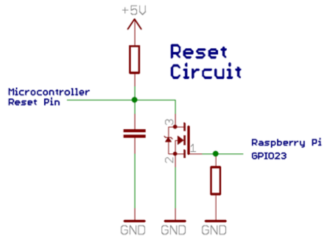
Abbildung 49: Prinzip-Schaltbild: Reset-Schaltung
