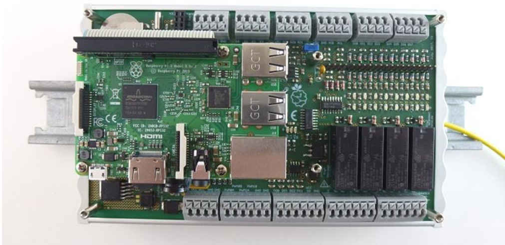
Abbildung 18: Hutschiene montage abgeschlossen
