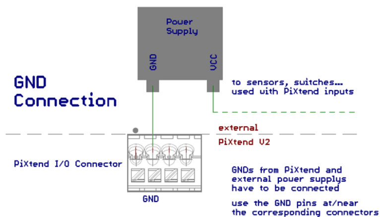
Abbildung 67: Prinzip-Schaltbild: GND-Verbindung
