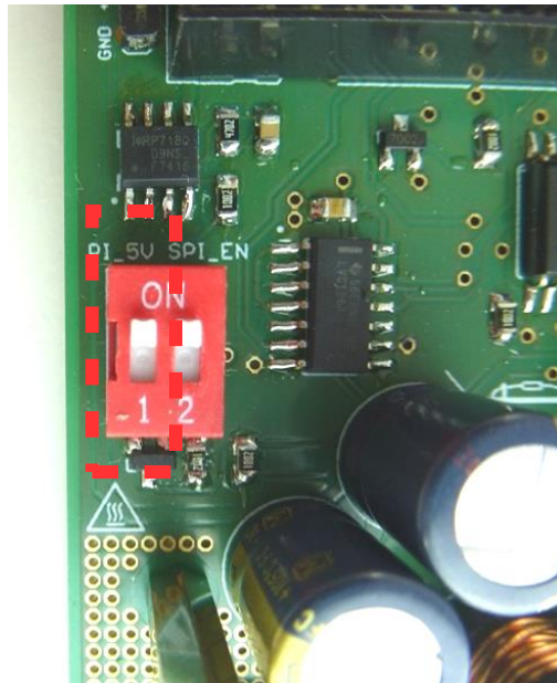
Abbildung 29: Schalter - „PI_5V“ in der Stellung „ON“
