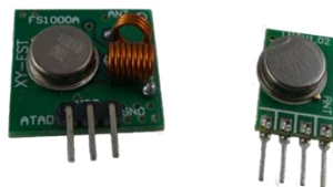
Abbildung 74: Typische „low-cost“ 433 MHz-Funktransmitter
