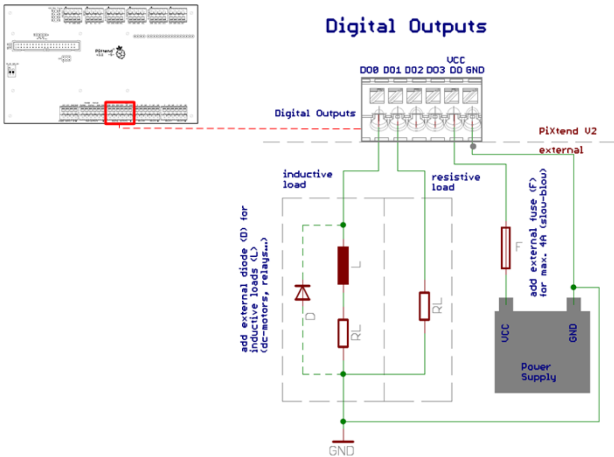
Abbildung 56: Prinzip-Schaltbild: Anschluss der digitalen Ausgänge
