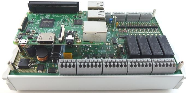
Abbildung 14: Hutschienegehäuse montiert
