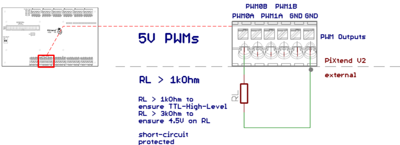
Abbildung 71: Prinzip-Schaltbild: Anschluss der PWM- bzw. Servo-Ausgänge
