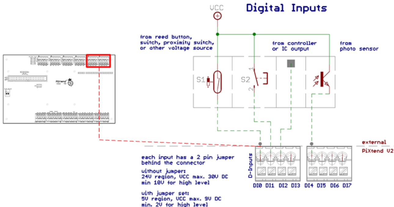
Abbildung 53: Prinzip-Schaltbild: Anschluss der digitalen Eingänge
