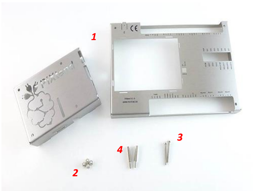
Abbildung 3.1: Lieferumfang – Edelstahlhaube (Artikelnummer 30199 007)
