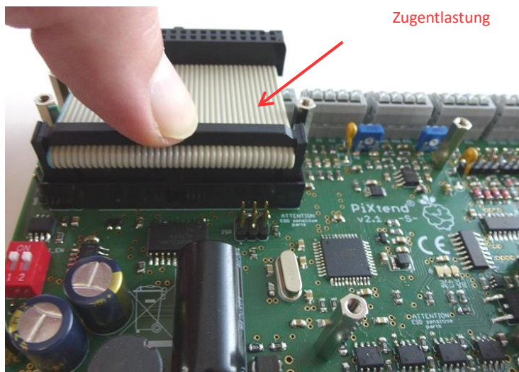
Abbildung 6: Flachbandkabel auf PiXtend V2 -S- stecken
