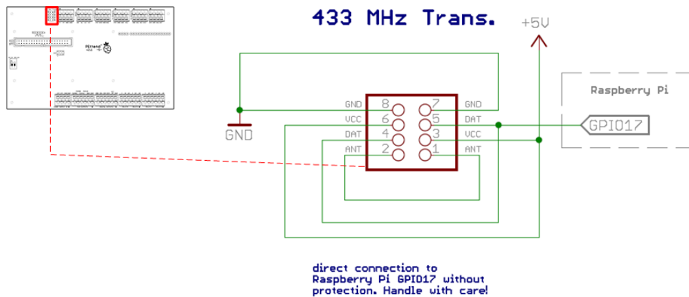
Abbildung 75: Prinzip-Schaltbild: Anschluss von 433 MHz-Transmittern
