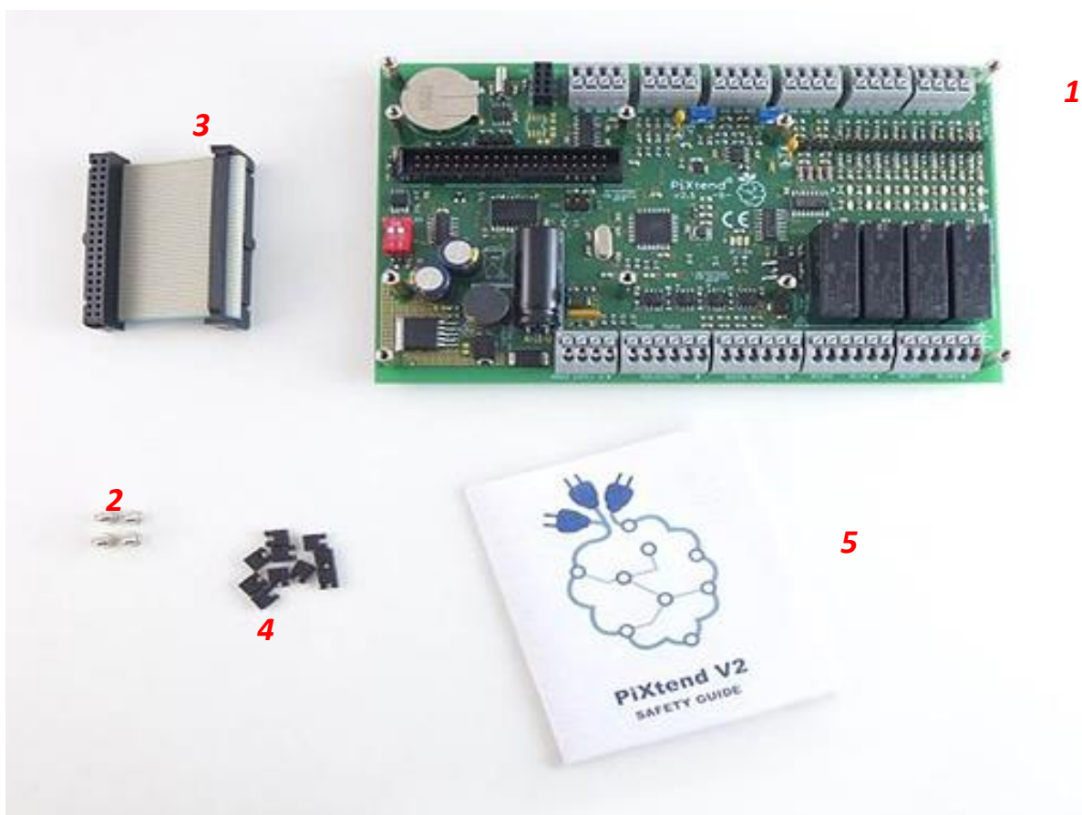
Abbildung 1: Lieferumfang - PiXtend V2 -S- Extension Board (Artikelnummer 50199 004)
