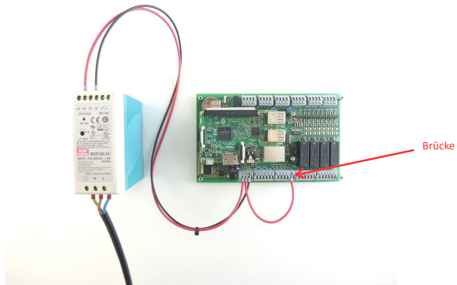
Abbildung 37: 24V; 2,5 A Hutschienennetzteil an PiXtend angeschlossen
