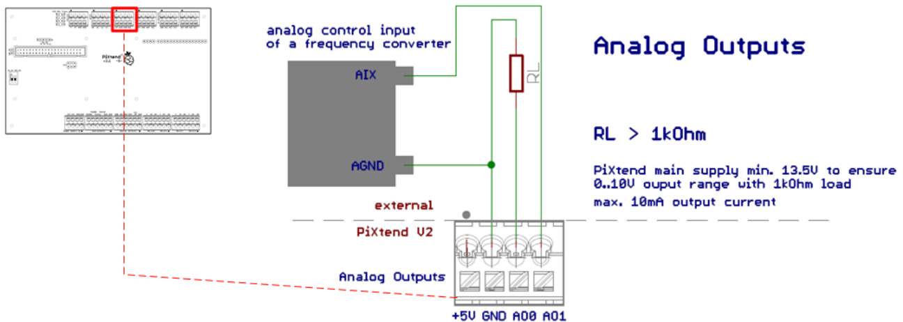
Abbildung 69: Prinzip-Schaltbild: Anschluss der analogen Spannungsausgänge
