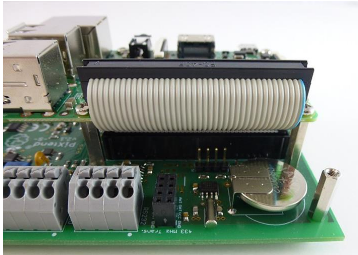
Abbildung 41: Verbindung zwischen PiXtend V2 -S- und Raspberry Pi
