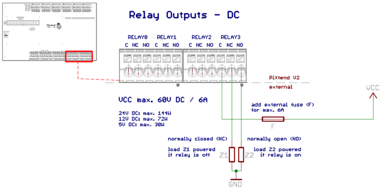
Abbildung 58: Prinzip-Schaltbild: Anschluss der Relais (Gleichspannung)
