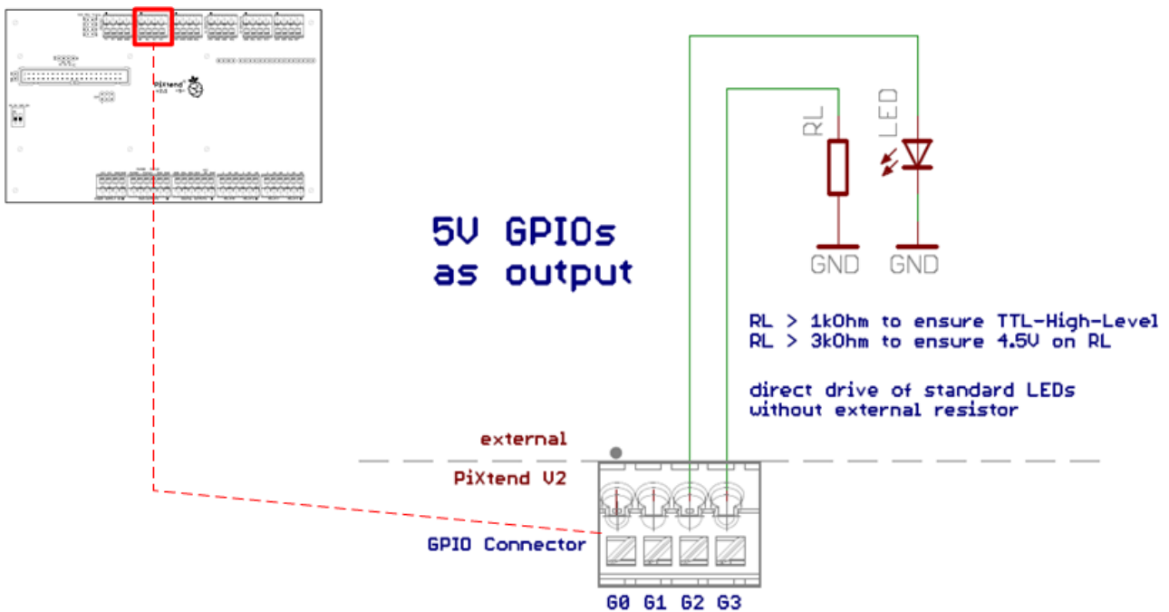
Abbildung 62: Prinzip-Schaltbild: Anschluss der GPIOs (als Ausgänge)
