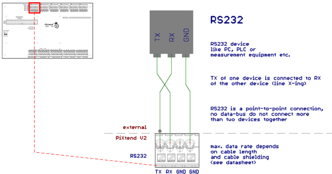
Abbildung 77: Prinzip-Schaltbild: Anschluss der RS232-Schnittstelle
