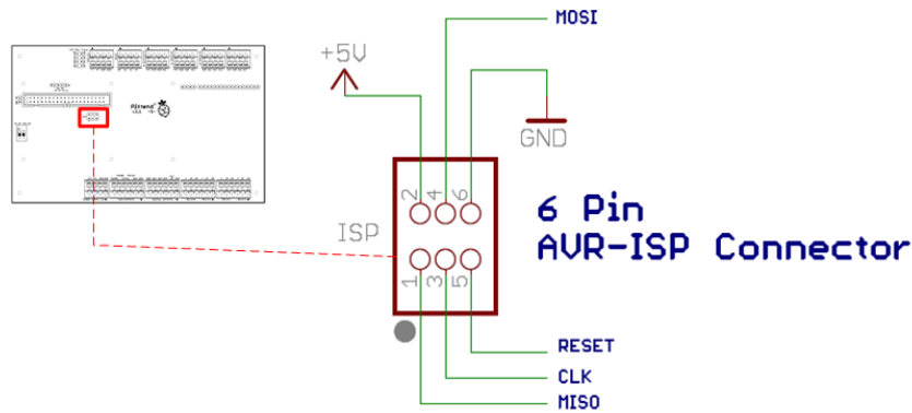
Abbildung 51: Prinzip-Schaltbild: Anschluss eines Programmieradapters
