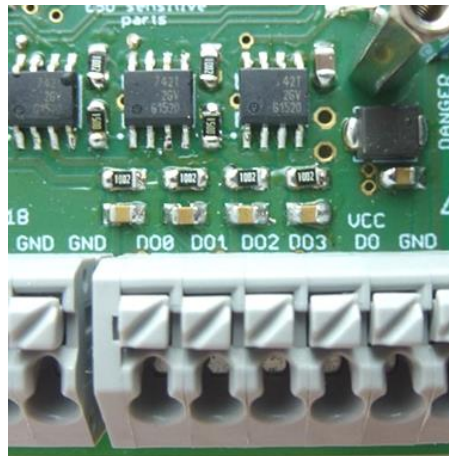
Abbildung 55: Anschlussleiste - digitale Ausgänge
