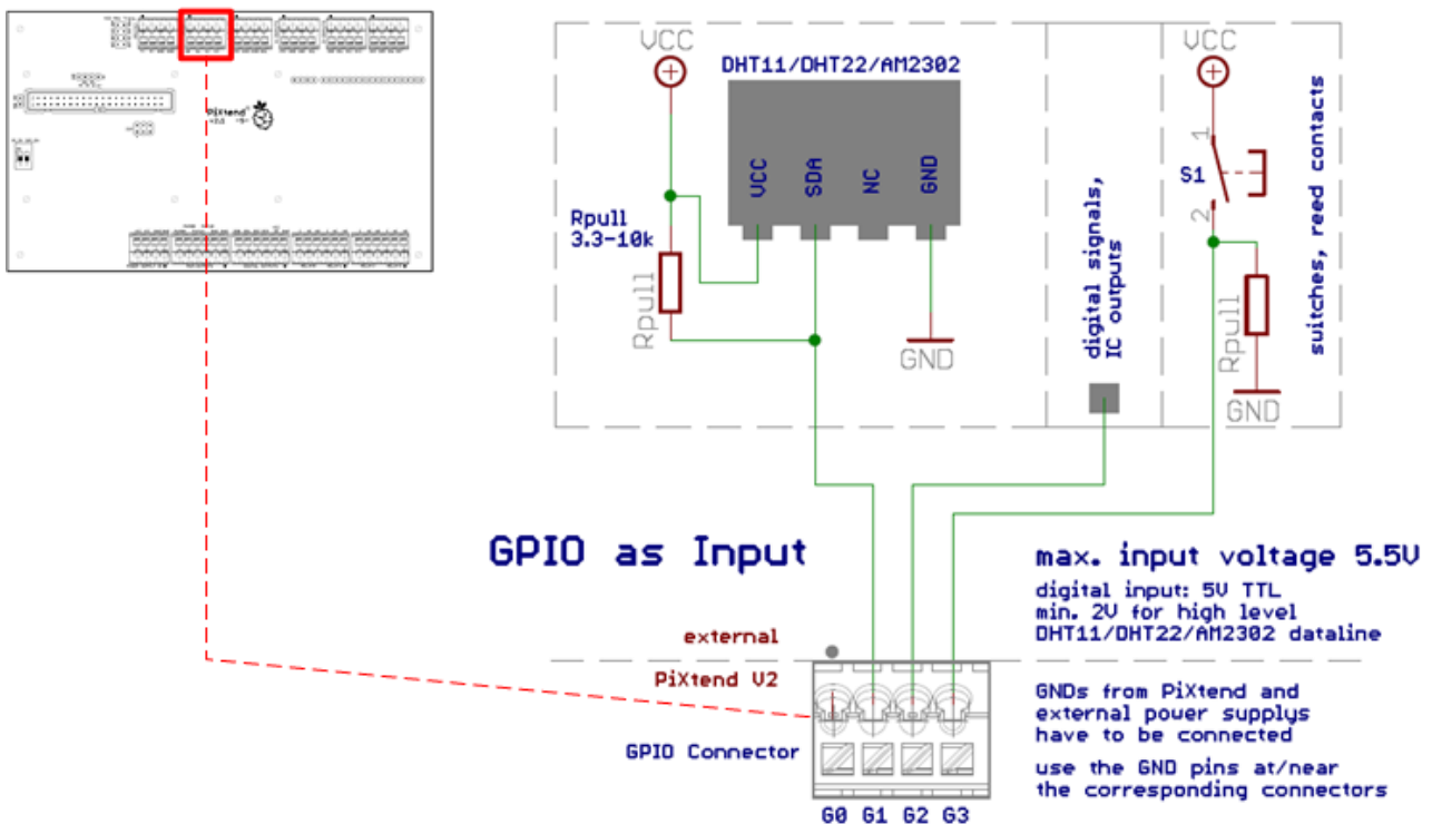
Abbildung 61: Prinzip-Schaltbild: Anschluss der PiXtend V2 -S- GPIOs (als Eingänge)
