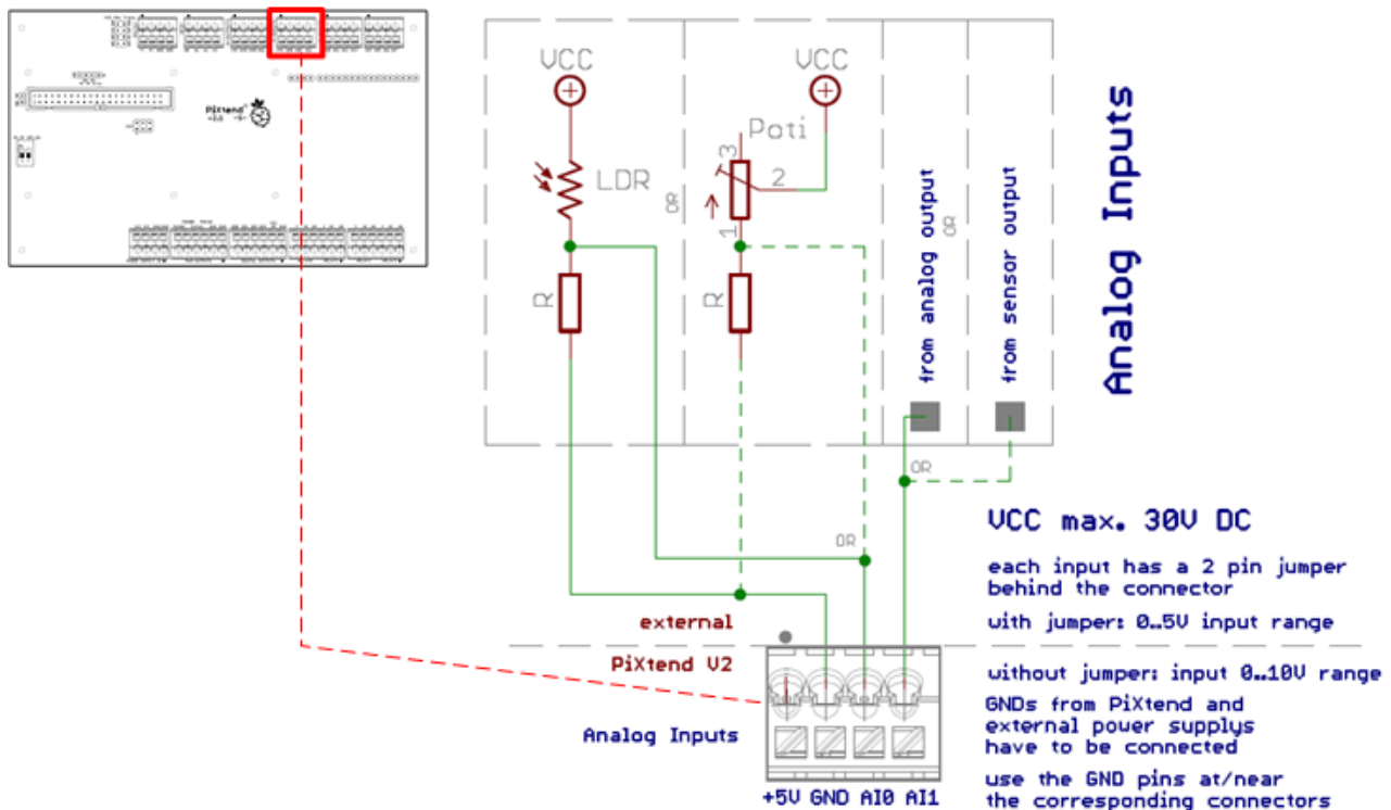
Abbildung 65: Prinzip-Schaltbild: Anschluss der analogen Spannungseingänge
