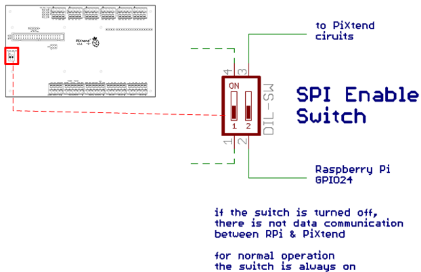
Abbildung 50: Prinzip-Schaltbild: SPI-Enable
