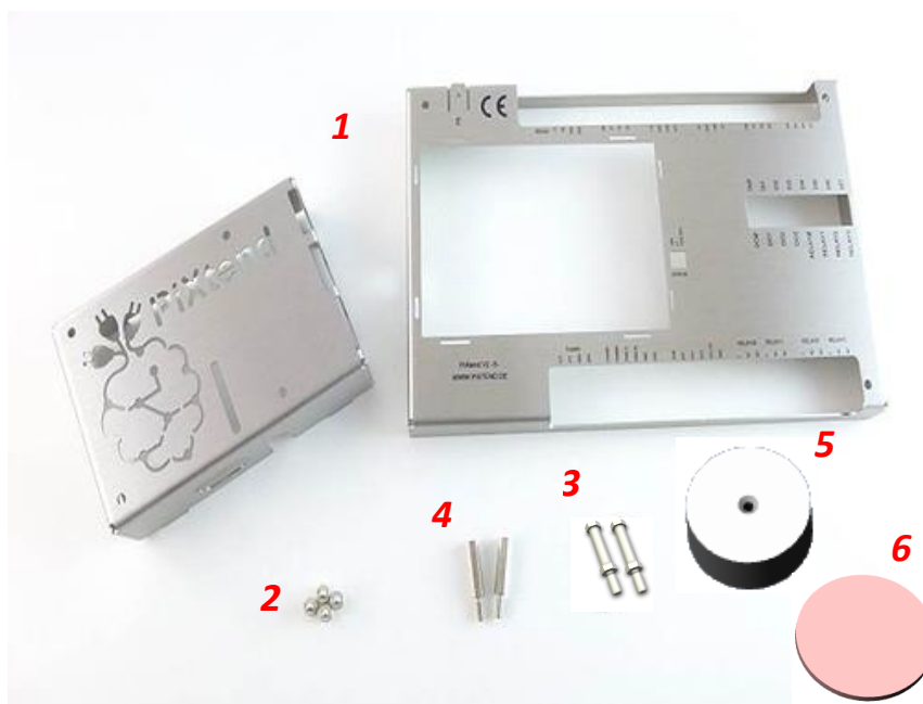
Abbildung 3.2: Lieferumfang – Edelstahlhaube Pi4 (Artikelnummer 30199 013)
