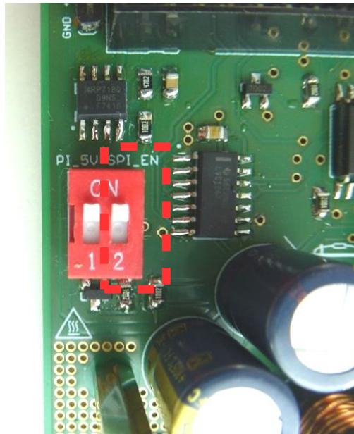
Abbildung 47: DIP-Schalter: SPI_EN
