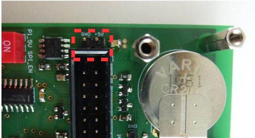
Abbildung 45: Versorgungsanschluss - Raspberry Pi 7" Touch-Display
