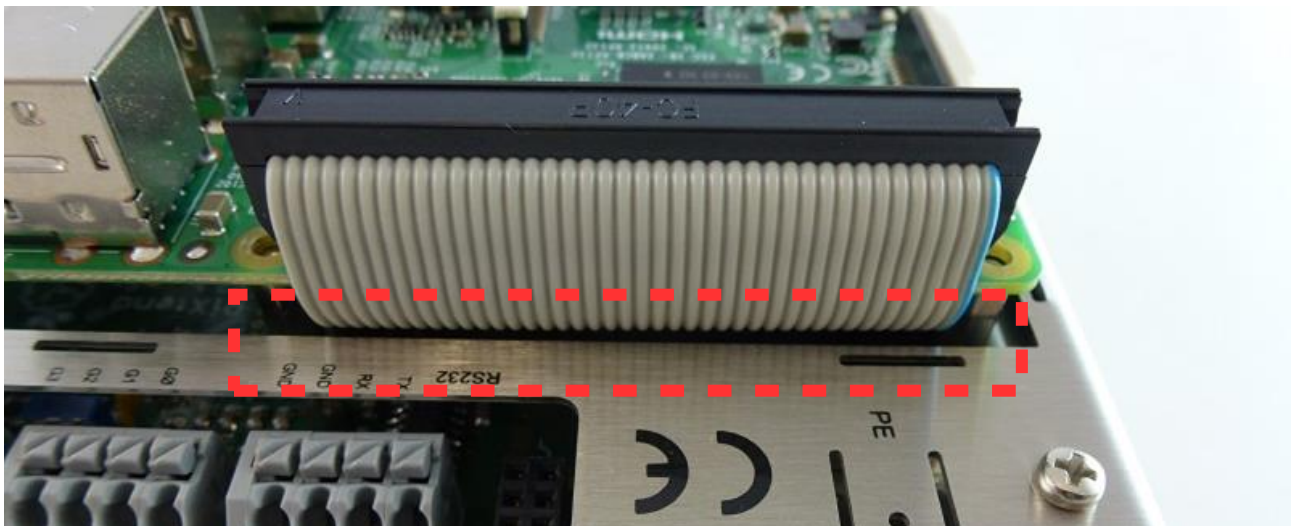
Abbildung 24: Sicherheitsabstand zwischen Flachbandkabel und Haube
