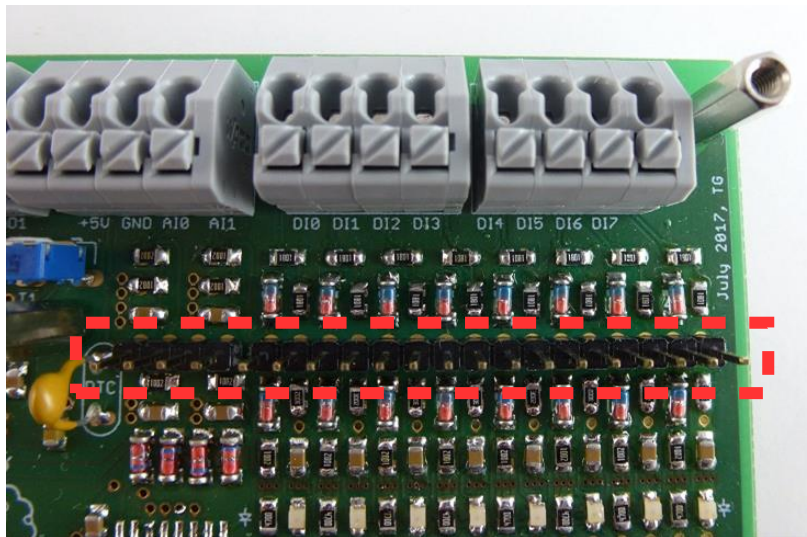
Abbildung 31: Jumper - digitale Eingänge im 24V Bereich (Werkseinstellung)
