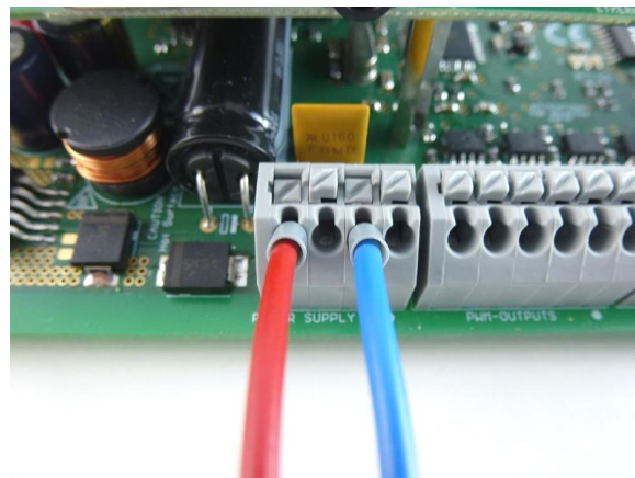
Abbildung 35: Versorgungsanschluss auf PiXtend V2 -S-
