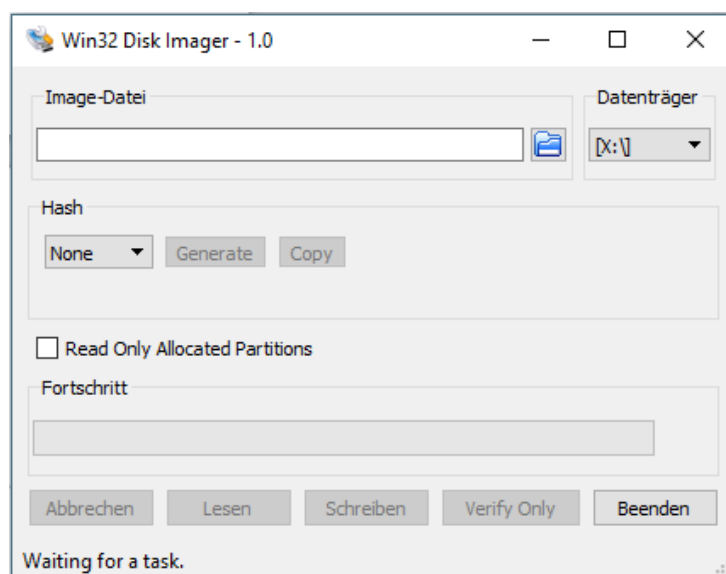
Abbildung 32: Software - Win32DiskImager
