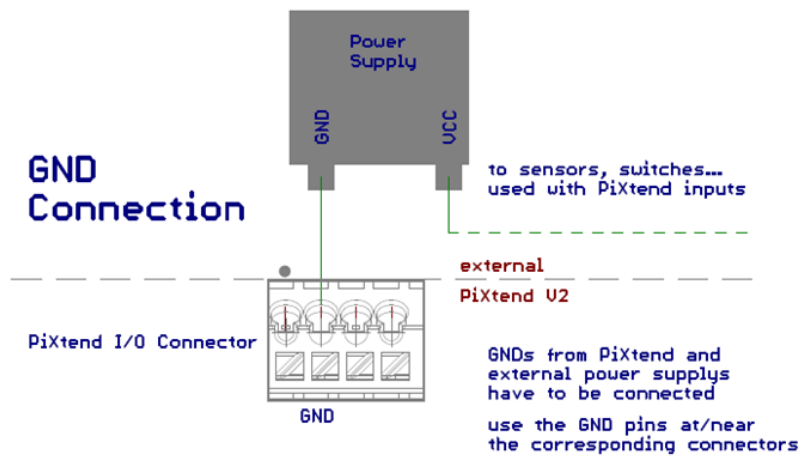
Abbildung 54: Prinzip-Schaltbild: GND-Verbindung
