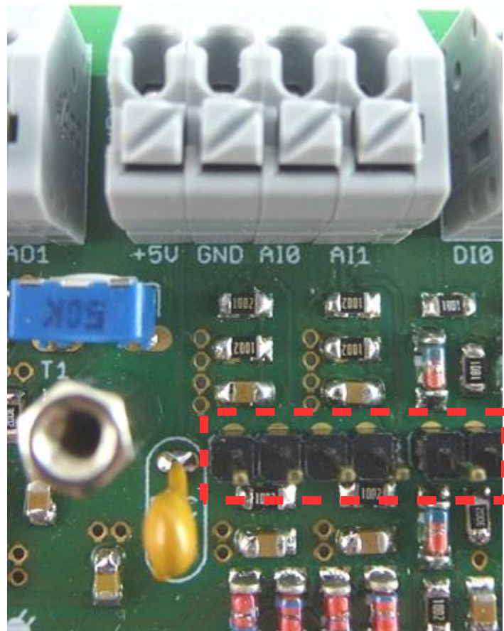
Abbildung 30: Jumper - analoge Spannungseingänge im 10V Messbereich (Werkseinstellung)
