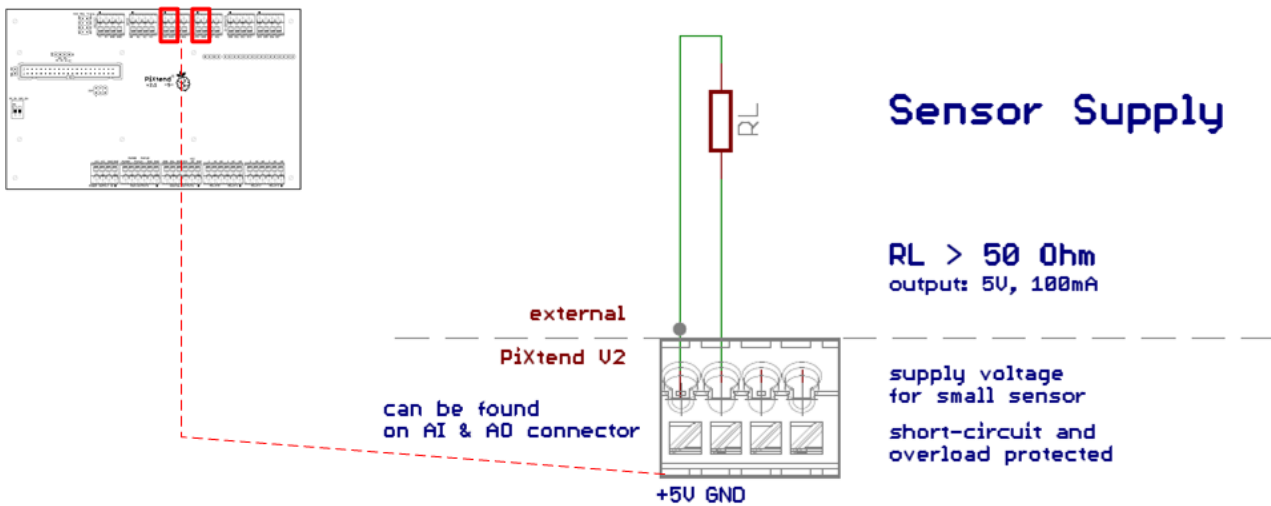
Abbildung 66: Prinzip-Schaltbild: Anschluss der Sensorversorgung
