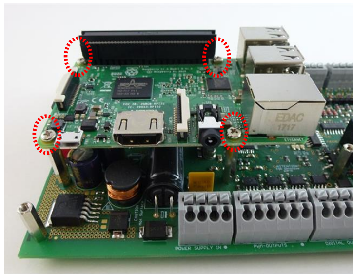
Abbildung 8: Raspberry Pi auf PiXtend V2 -S- verschrauben
