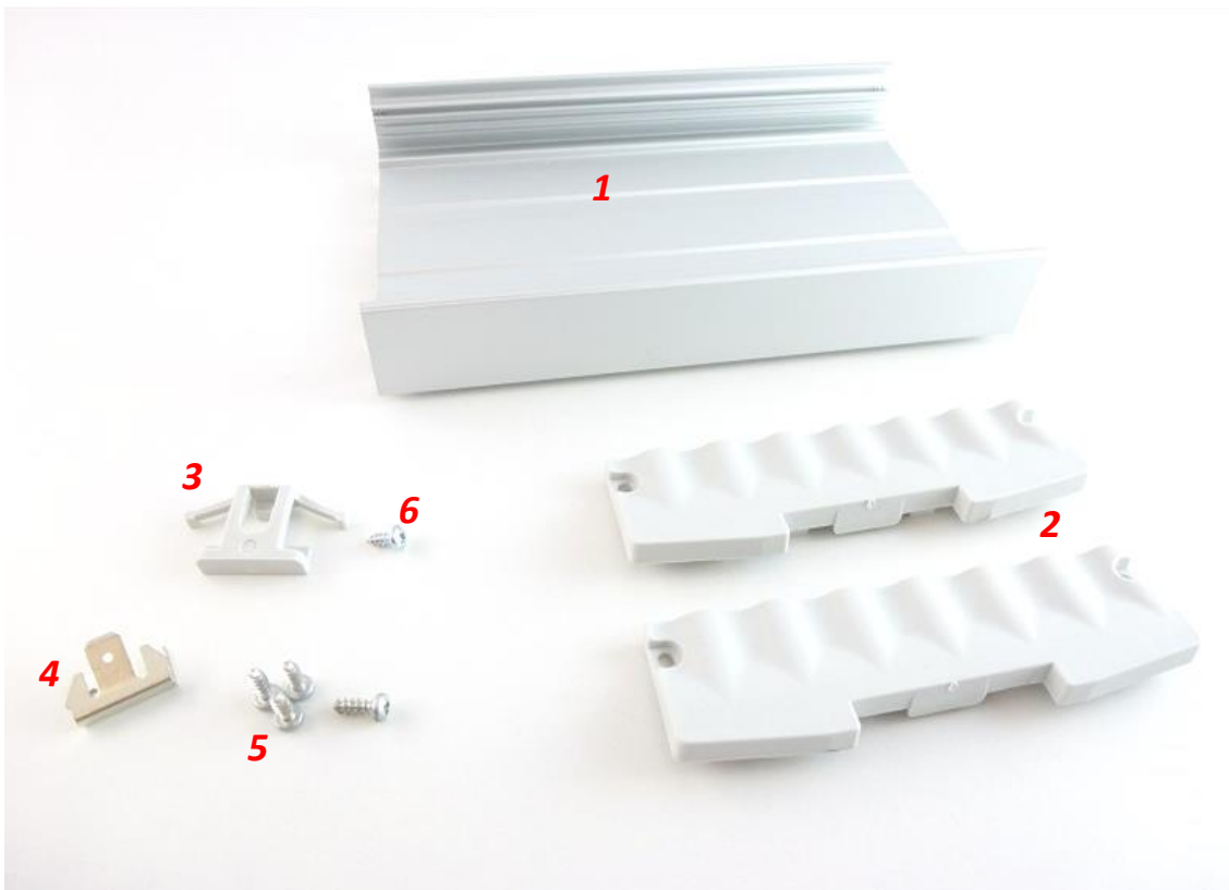
Abbildung 2: Lieferumfang – Hutschienengehäuse (Artikelnummer 30199 008)
